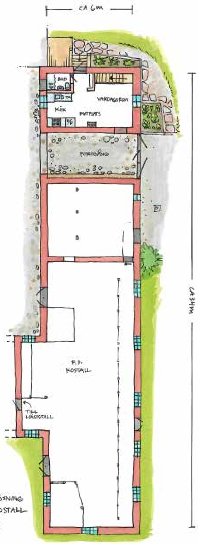
UNGEFÄRLIG PLANLÖSNING OVANVÅNING ~ LÄGENHET GYLLE 10:12
